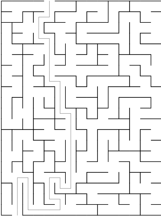
Maze 93
